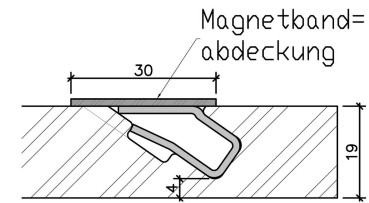
Querschnitt
